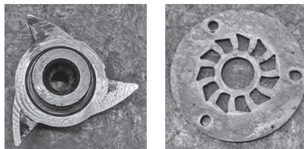
Рис. 21 Профессиональный режущий механизм
