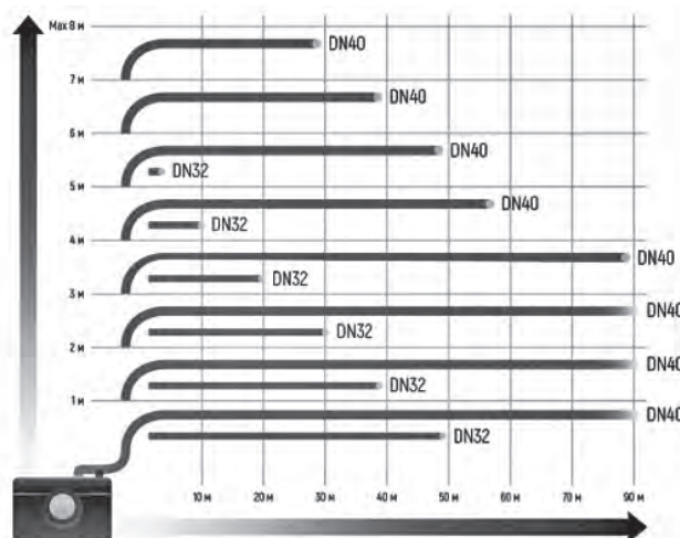
Рис. 23 Максимальная длина напорного трубопровода
