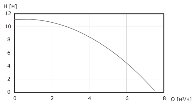
Рис. 24 Рабочие характеристики CITILIFT TRIO
