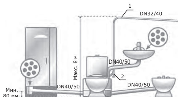
Рис. 22 Рекомендуемая схема монтажа напорного трубопровода
